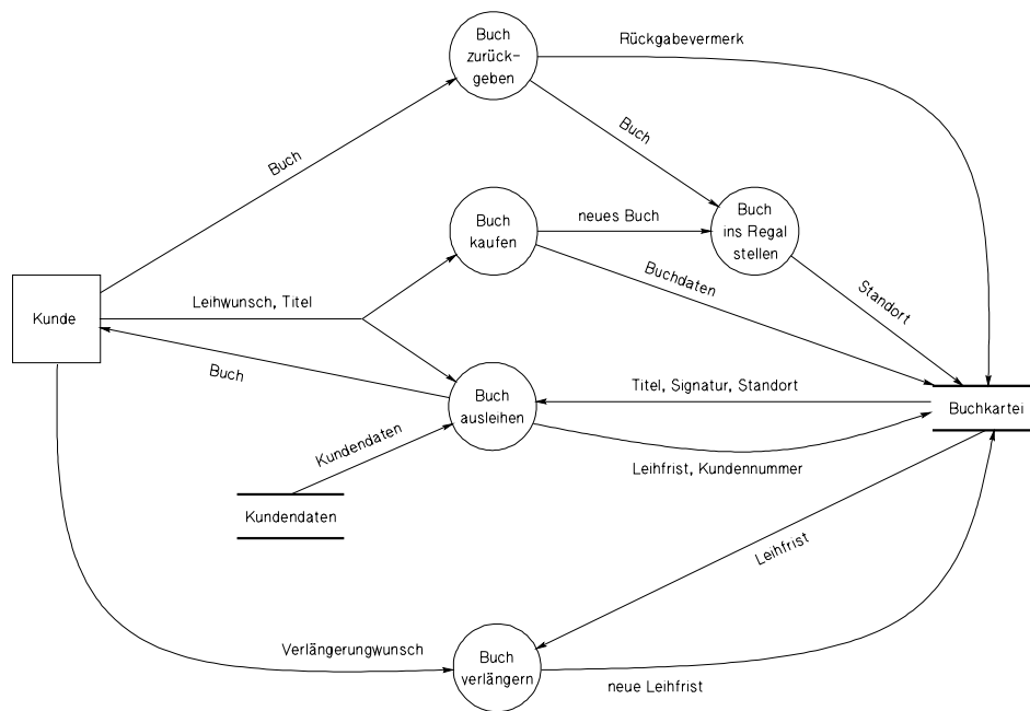
Abbildung 1: Daten-Fluß-Diagramm
