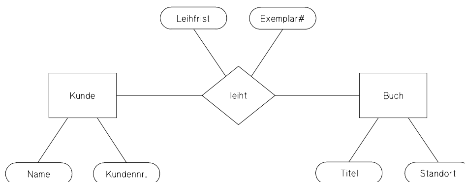
Abbildung 8: Entity-Relationship-Diagramm
