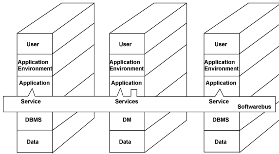
Abb. 1 OKIS software bus [28]
