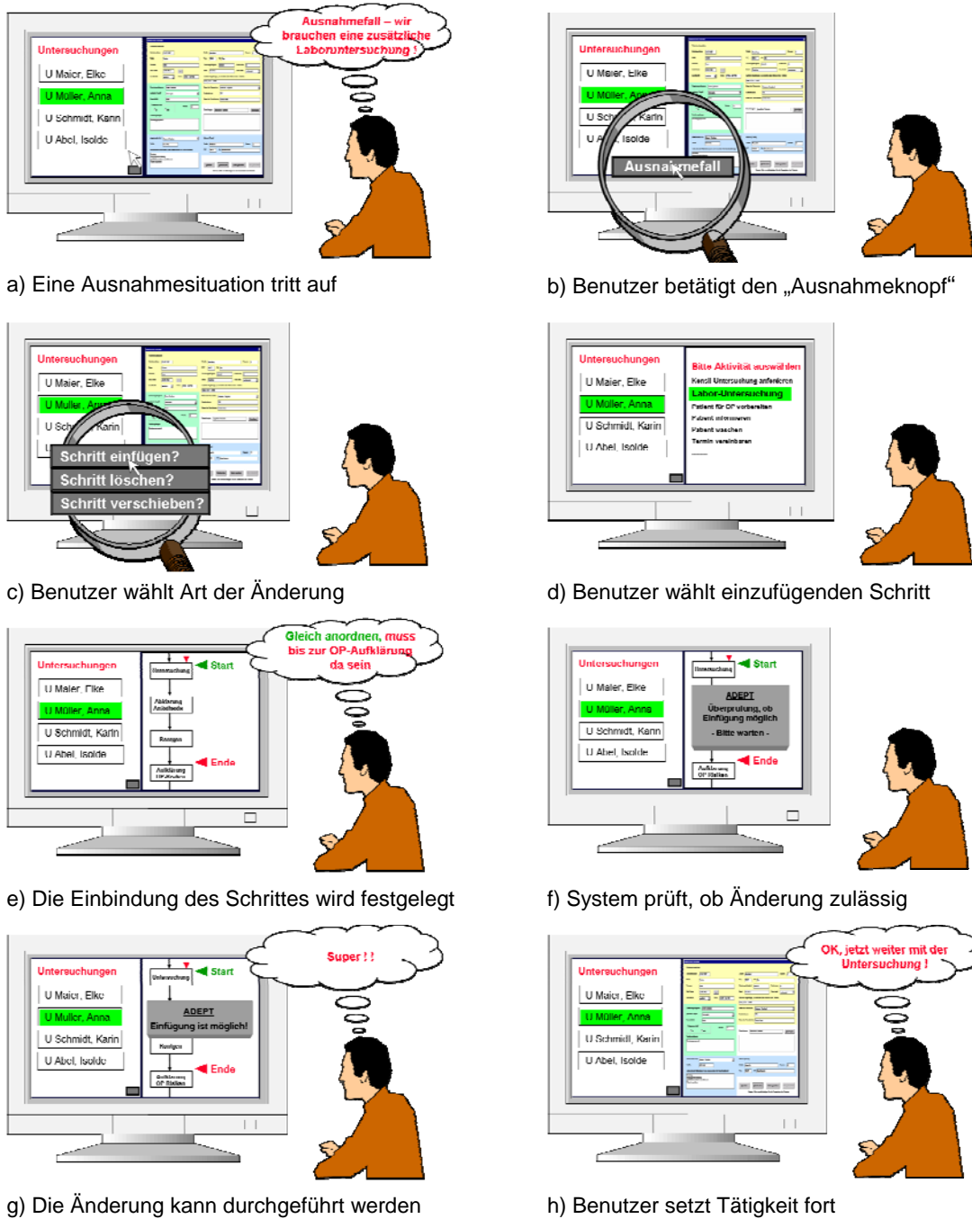
Abb. 5: Durchführung einer Ad-hoc-Abweichung aus Benutzersicht [Dada06]
