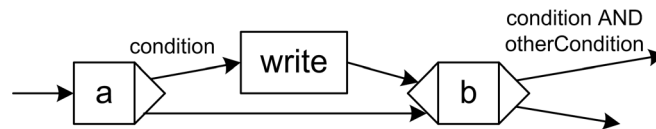
Abbildung 4-5: Ausschnitt aus einem Prozess, in dem nur unter bestimmten Bedingungen bestimmte externe Daten geschrieben werden (Aktivität „write“)
