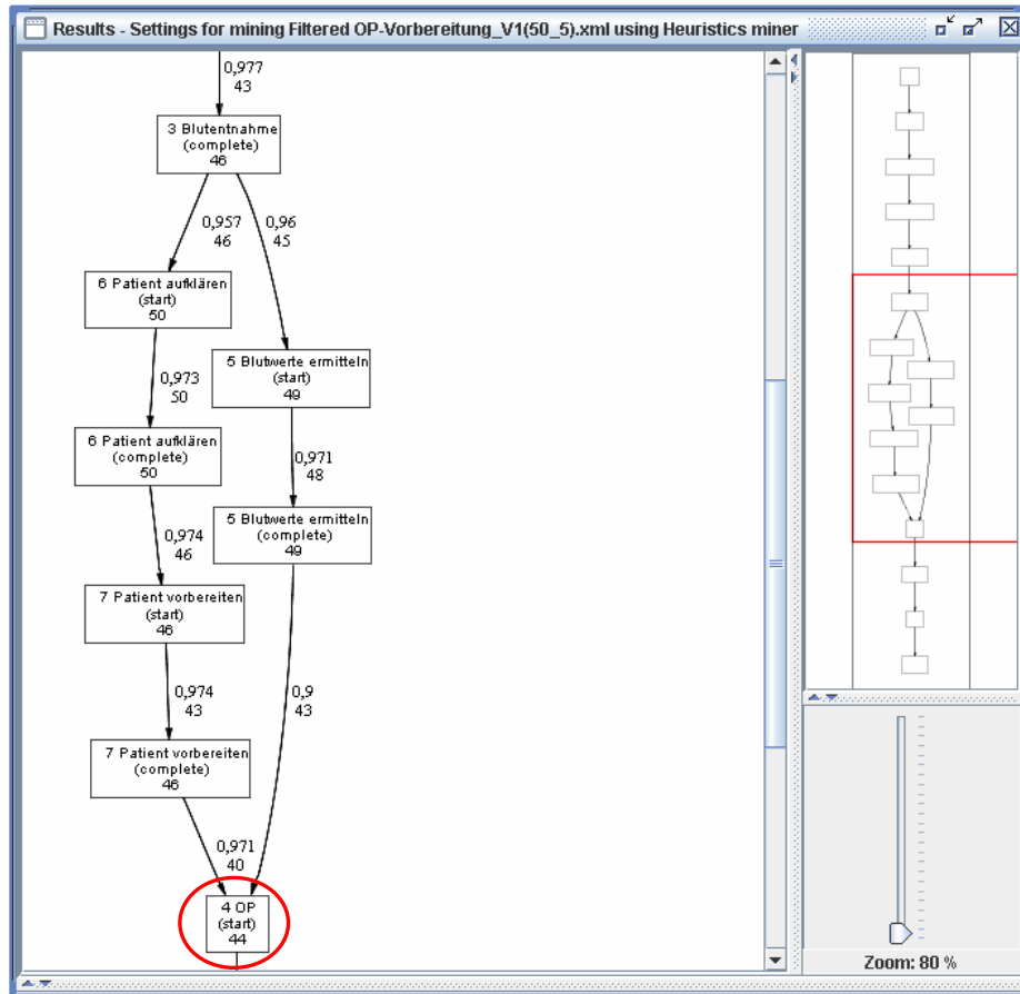
Abbildung 3-30: Beispiel Heuristics Miner: OP-Vorbereitung, V1, 50 Instanzen, 5 % einfache Noise
