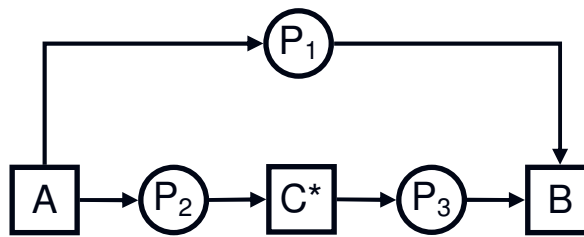
Abbildung 3-52: Implizite Abhängigkeit in einem Petrinetz [WWS06]
