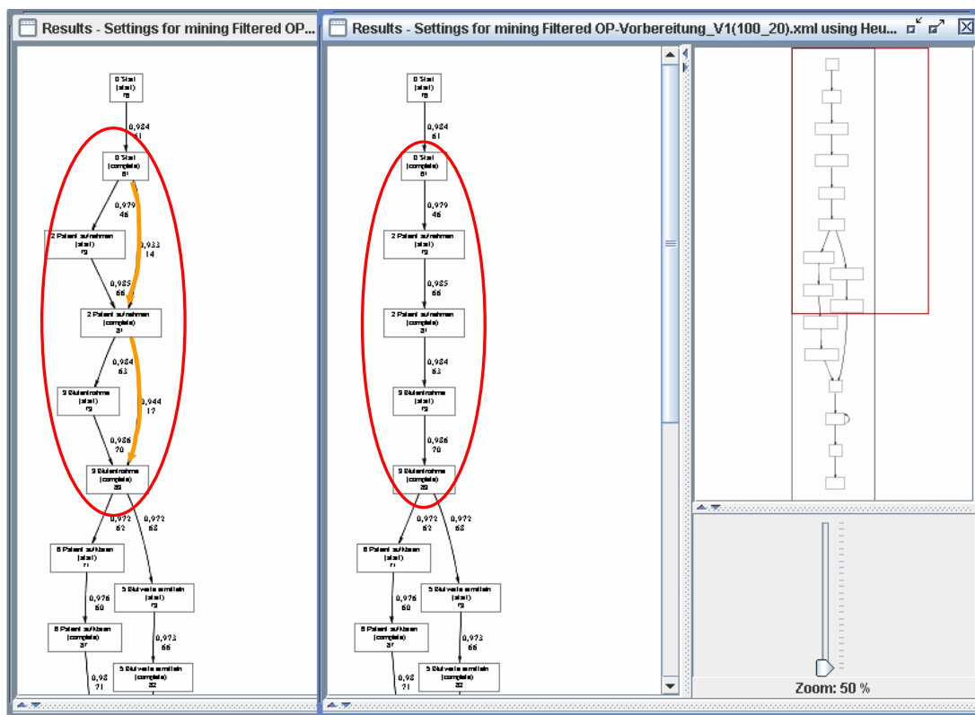
Abbildung 3-31: Beispiel Heuristics Miner: OP-Vorbereitung, V1, 100 Instanzen, 20 % einfache Noise
