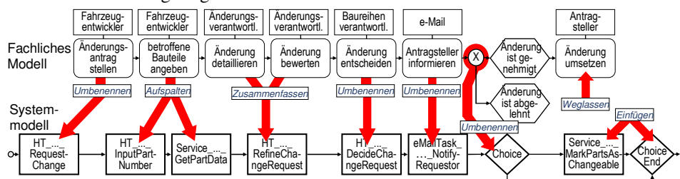
Abbildung 1: Transformationen zwischen fachlichem Modell und Systemmodell
