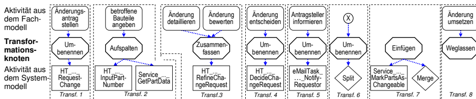
Abbildung 3: Abbildungsmodell für das in Abbildung 1 vorgestellte Beispielszenario
