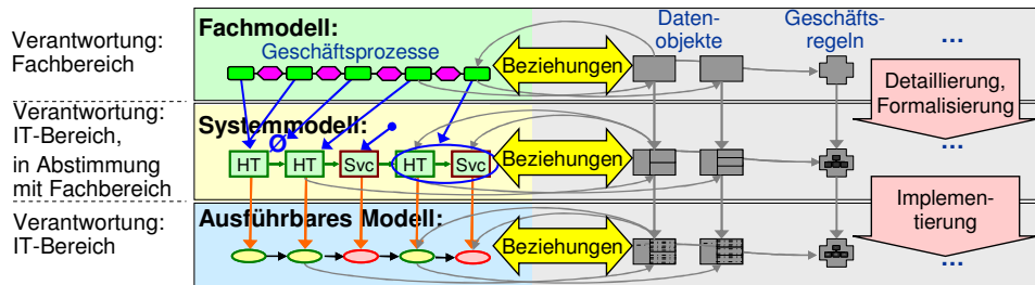
Abbildung 2: Ebenen der Modellierung von Prozessen und auch anderer Aspekte
